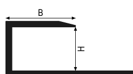
Alluminio B = 15 mm
