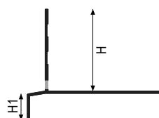
BD - Alluminio (Forato) H1 = 18 mm
