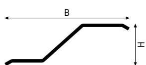
DK37 - Acciaio Inox - Ottone H = 12,5 mm Per spessori da 7 a 12,5 mm
