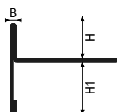
Alluminio B = 3,6 mm
