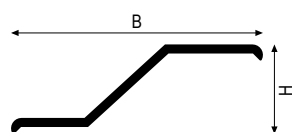
DK37 - Alluminio H = 12,5 mm
