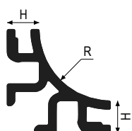
SB 10 - Alluminio R = 10 mm
