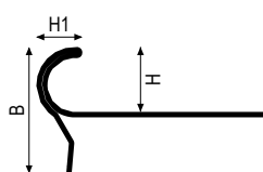
Acciaio Inox - FLR H1 = 8,5 mm
