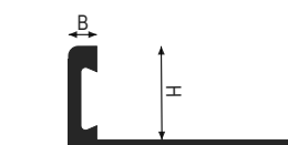
Alluminio TR 60 ÷ 150 B = 3 mm
