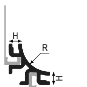
SB 10 + TR - Alluminio R = 10 mm
