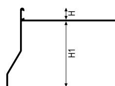
Alluminio BCS H = 12,5 mm
