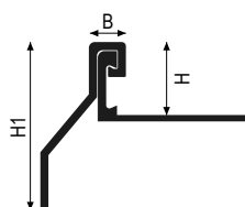
BTR 30 + TR - Alluminio
