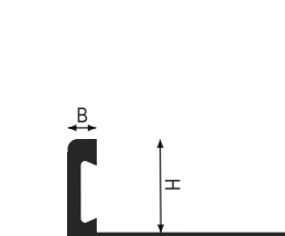
Resina Sintetica B = 3 mm
